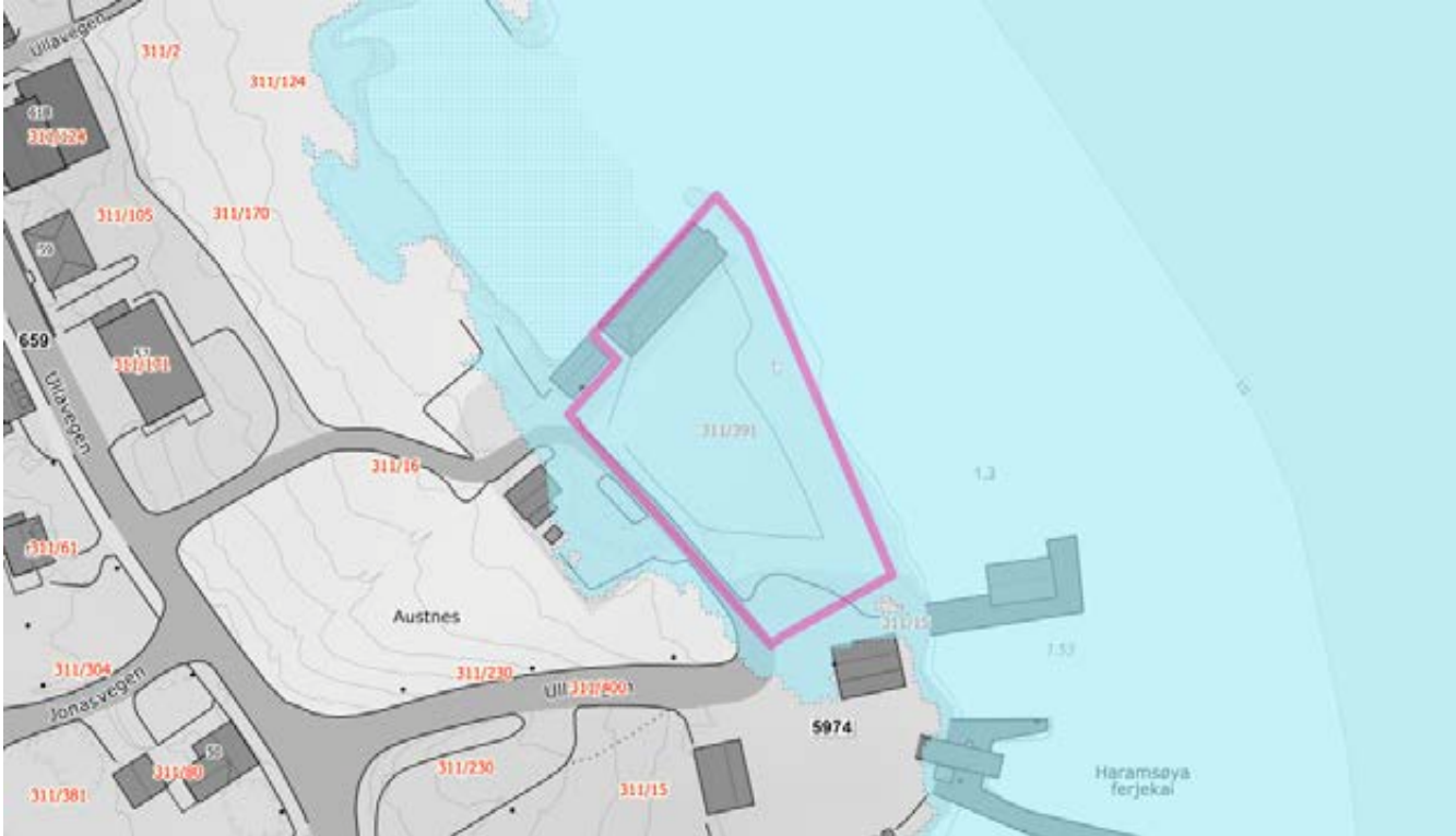
Middelhøyvann i år 2150
