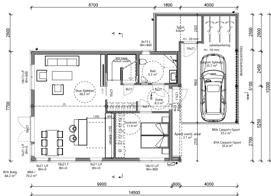
Plan 1. Etasje Bolig 2
