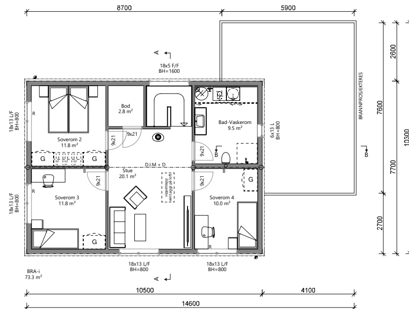
Plan 2. Etasje Bolig 2
