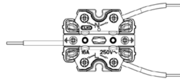
Koblings skjema
