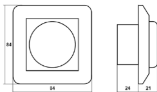
Målskisse
