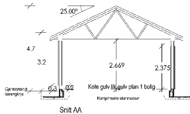
Snitt AA
