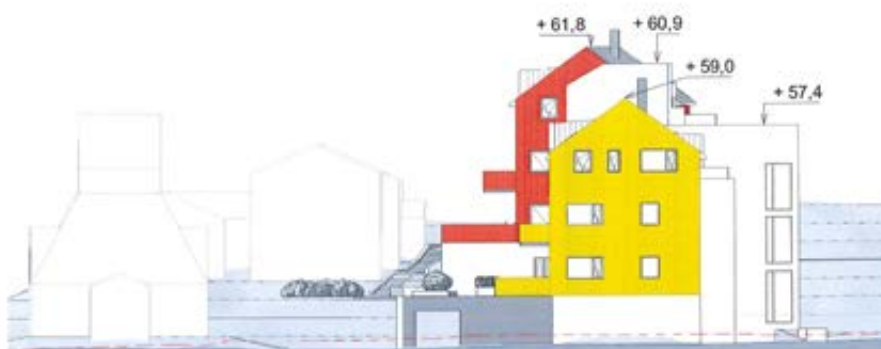
Fasade Øst 1 : 200
