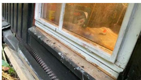
Vindu uten beslag på vannbrett
