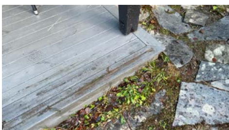
Værslitasje, konstruksjoner montert mot/nærme grunnen
