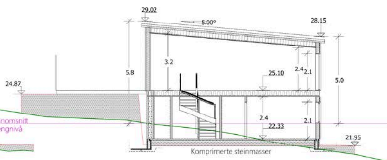
Snitt BB
