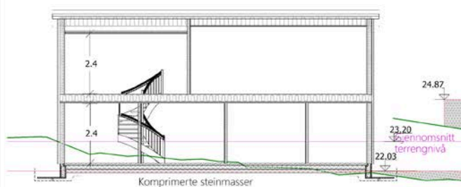
Snitt AA
