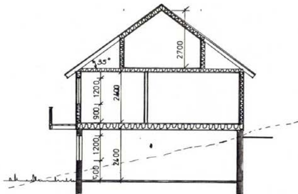
SNITT
