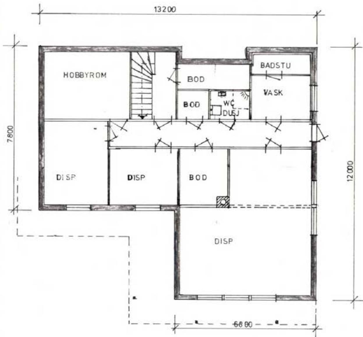
KJELLERPLAN
