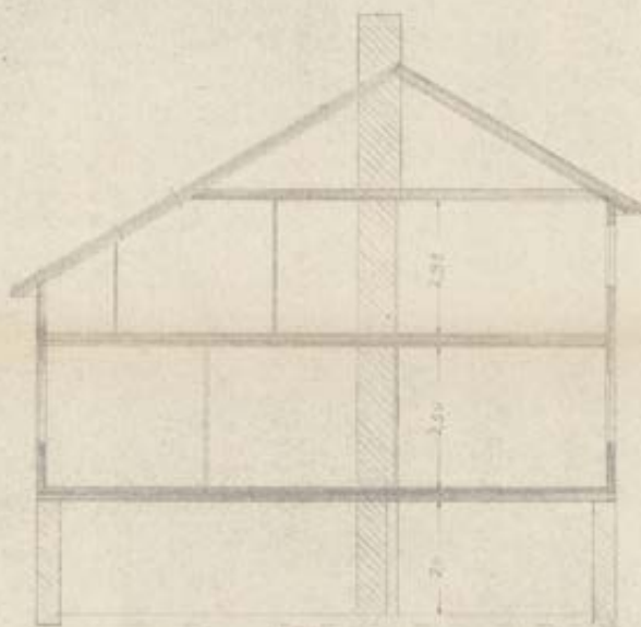
SNITT A-B
