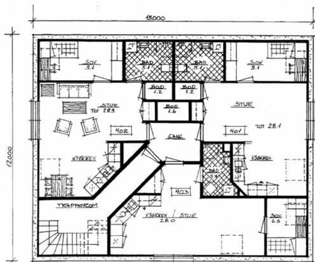
PLAN 4. ETG
