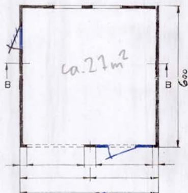
Plan Dobbel-garasje
