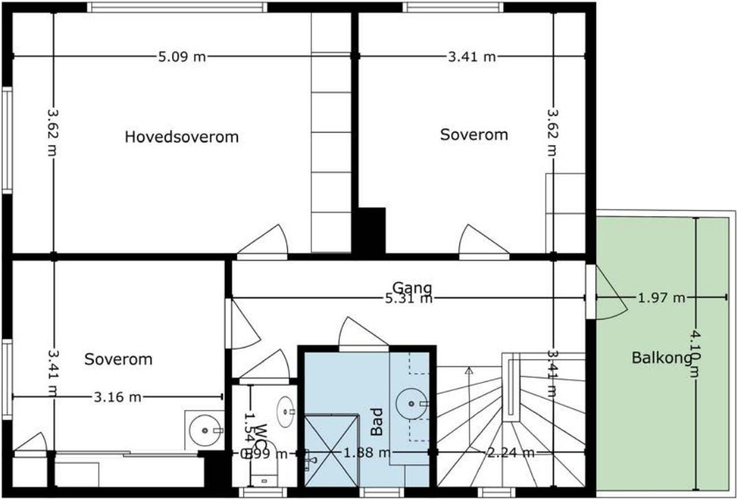
2. Etasje
