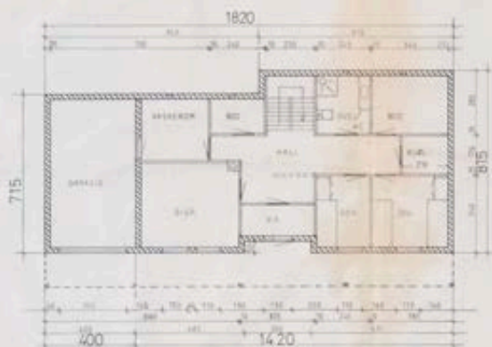
PLAN 801
