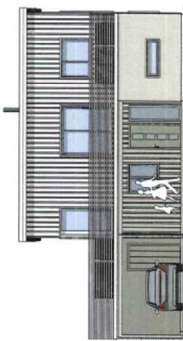
Fasade Sør 1:100
