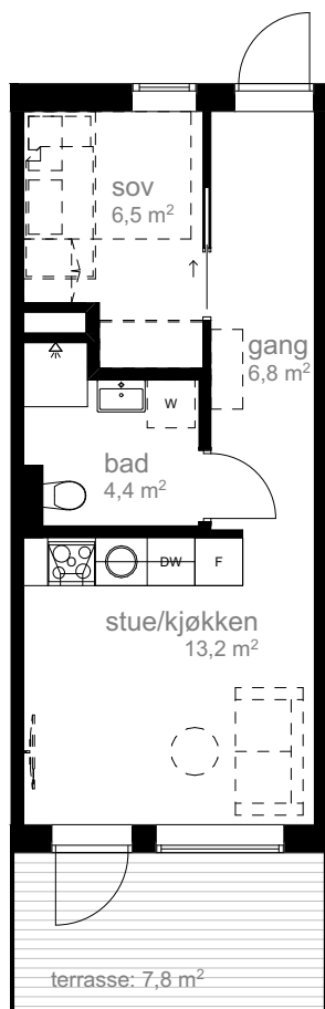
1. etasje 1:100
