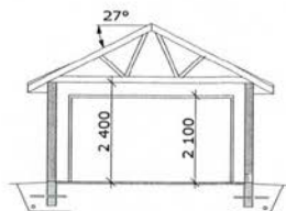
SNITT A-A
