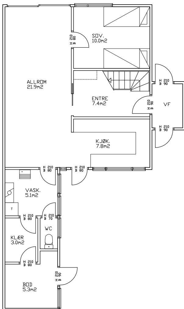
1. ETG.
