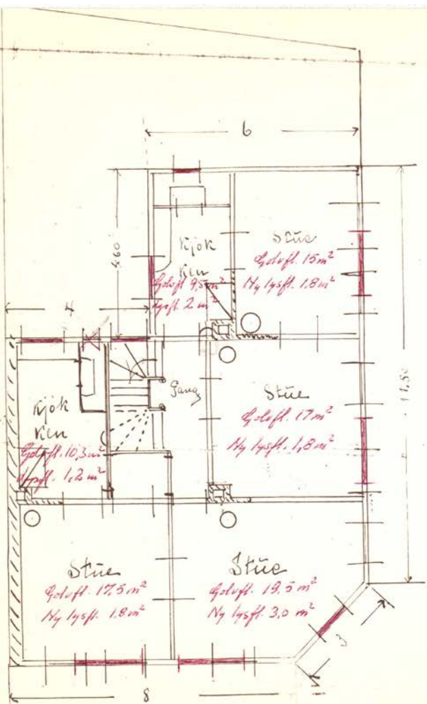
Situationsplan og 1/200 Etagesplan
