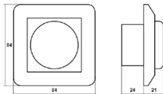
Målskisse
