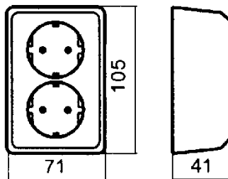
Målskisse
