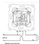
Koblingsskjema
