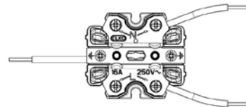
Koblingsskjema
