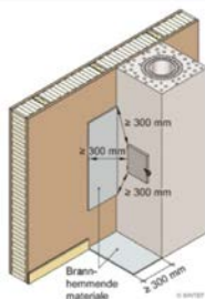
Fig. 43 Avstand fra feieluke eller sotluke til brennbart materiale, og anbefalt beskyttelse av gulv
