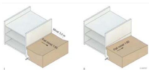
Fig. 32 a Avledning av vann på terreng I. Fall ut fra bygningen II. Fall langs bygningen
