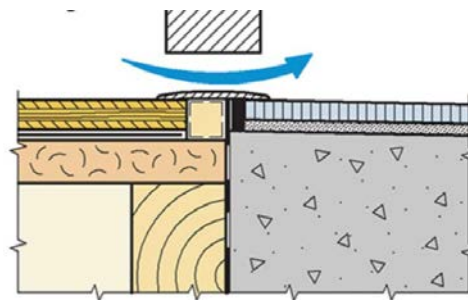
Prinsippskisse, overstrømming under døren. Kilde: Sintef.
