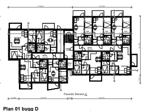
Plan 01 bygg D
