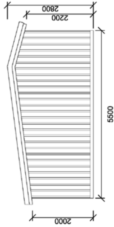
FASADE MOT ØST
