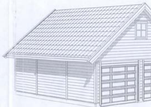
Perspektiv
