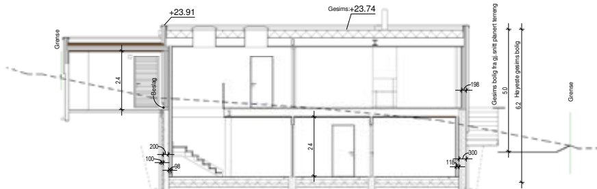
Snitt B-B
