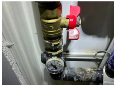
Lekkasje fra kobling i rør i rør skap.
