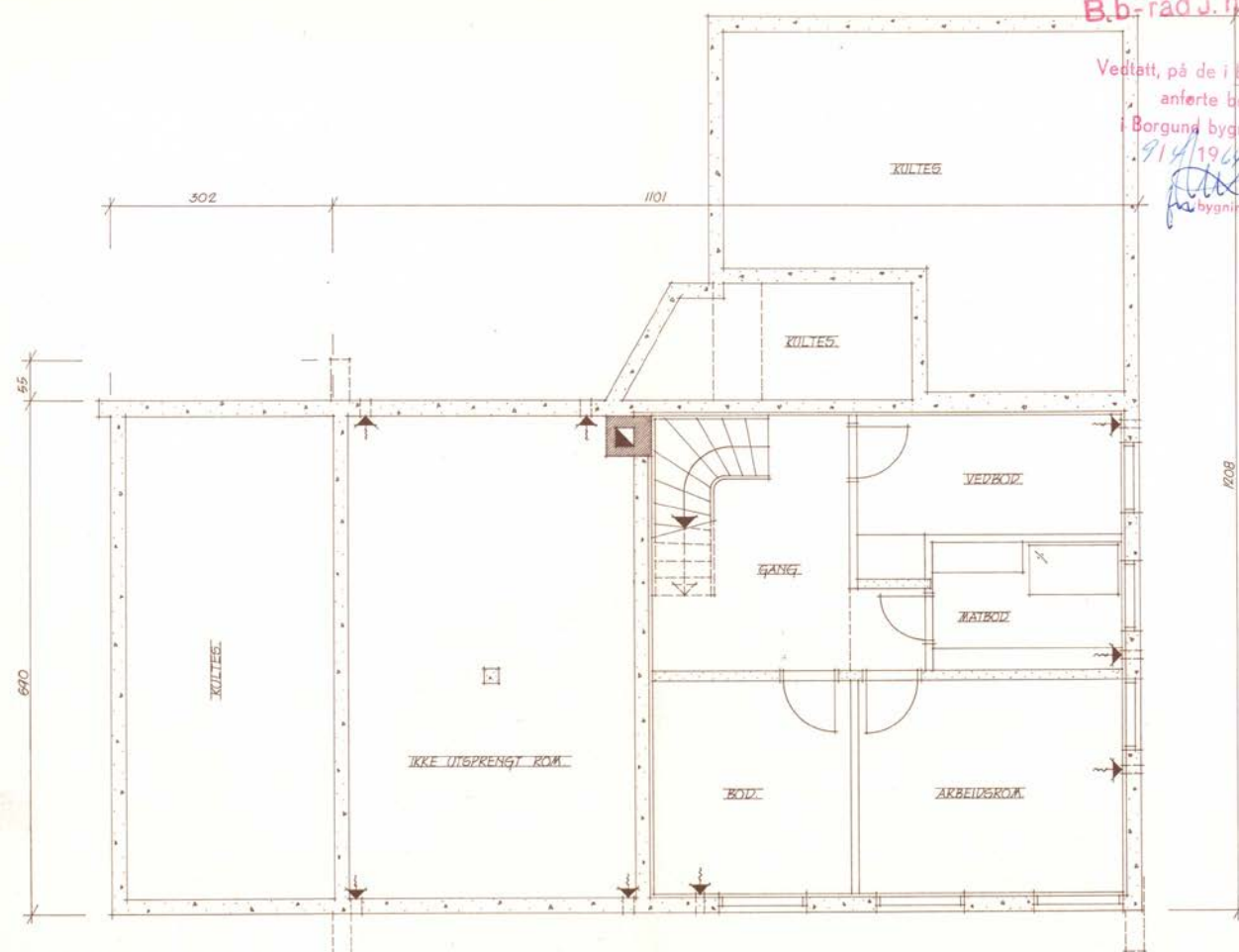
PLAN AV KJELLER - 1:50
