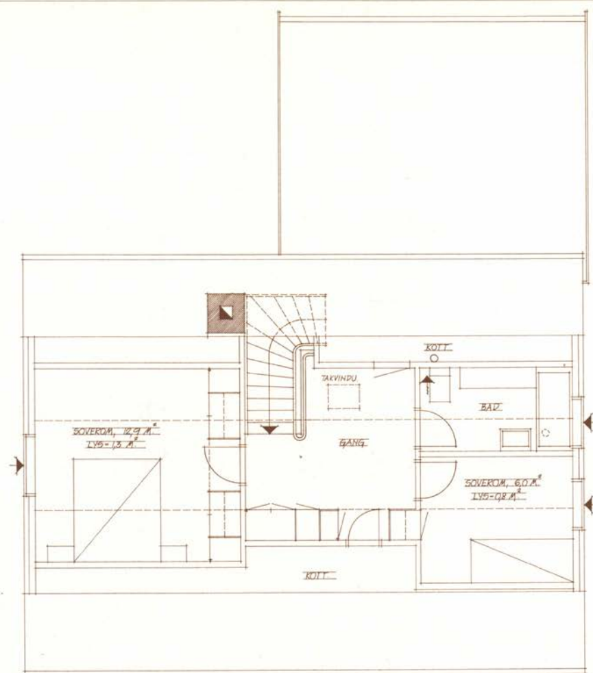
PLAN AV LOFT - M = 1:50
