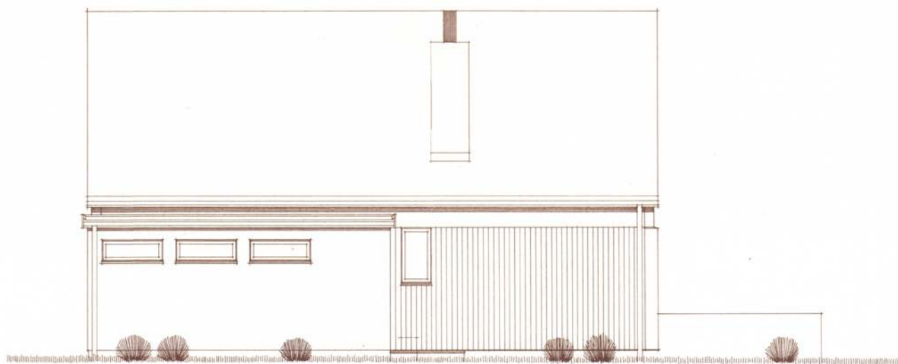
FASADE MOT NORD - MÅL = 1:50
