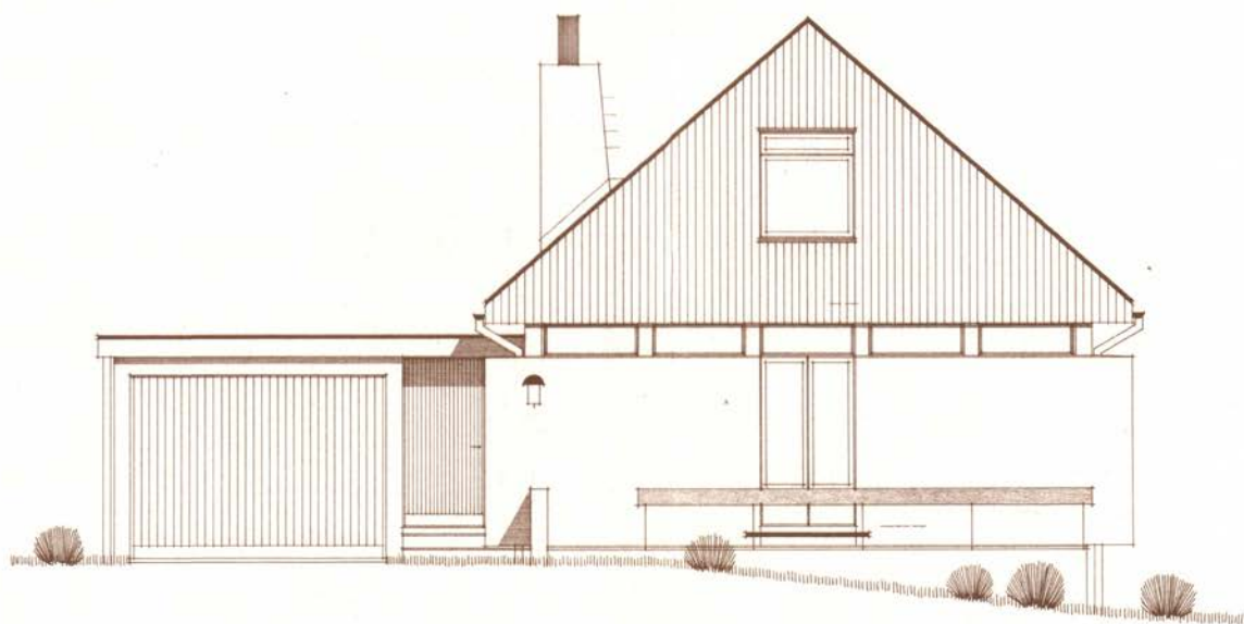
FASADE MOT VEST - MÅL - 1:50
