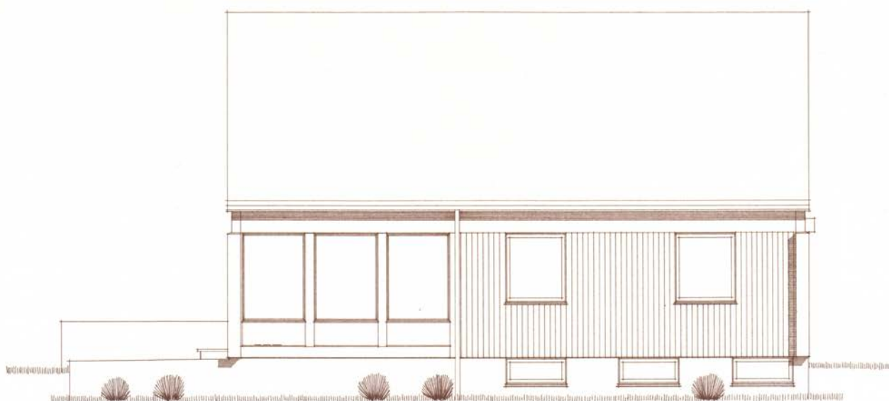
FASADE MOT SYD — MÅL — 1:50
