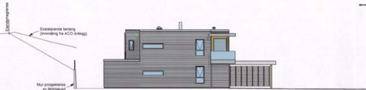
Fasade sør
